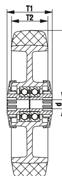
kuglični ležaj (CC) XKA izvedba
